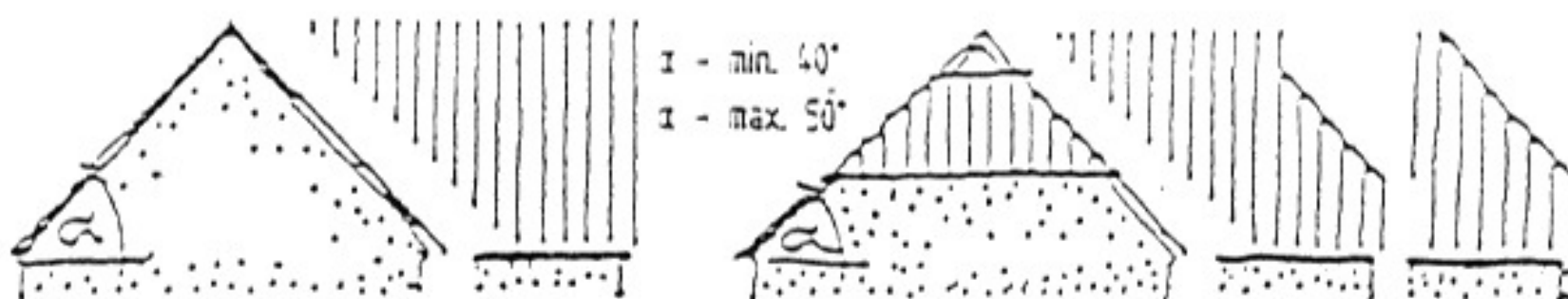
Satteldach und Krüppelwalmdach sind vorgeschrieben, Neigung zwischen 40-50°
