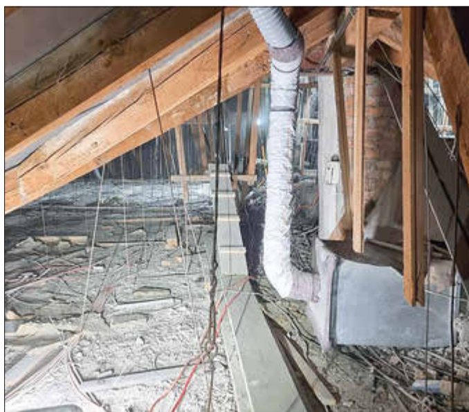
Dachtragwerk Rabitzdecke mit Abhängung an hunderten Seilen
