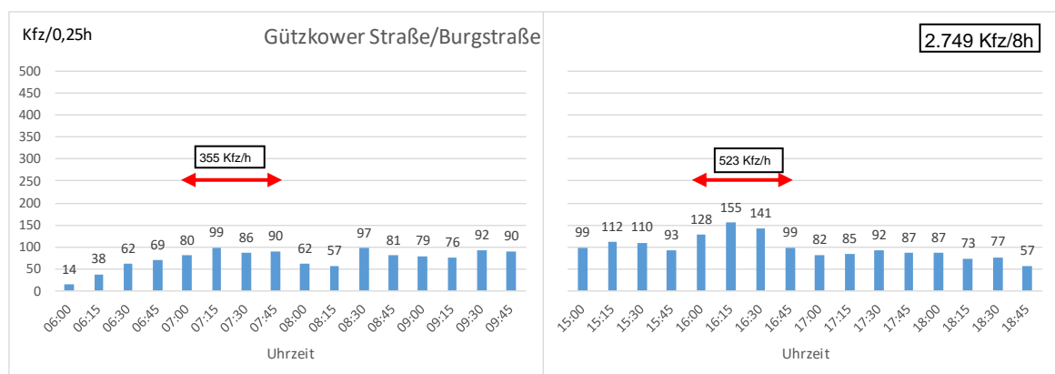
Abbildung 9 Tagesganglinie KP5 Gützkower Straße/Burgstraße Hochrechnung Durchschnittliche tägliche Verkehrsstärke (DTV)
