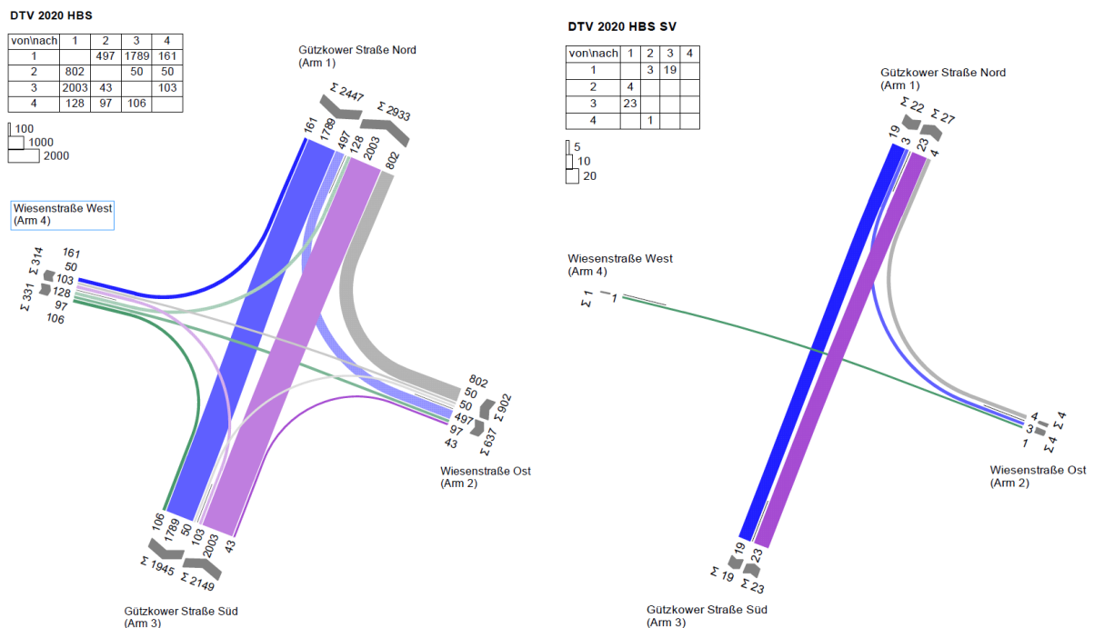
Abbildung 15 KP4 Gützkower Straße/Wiesenstraße DTV und DTV SV [Kfz/24h] DTV links, DTV SV rechts
