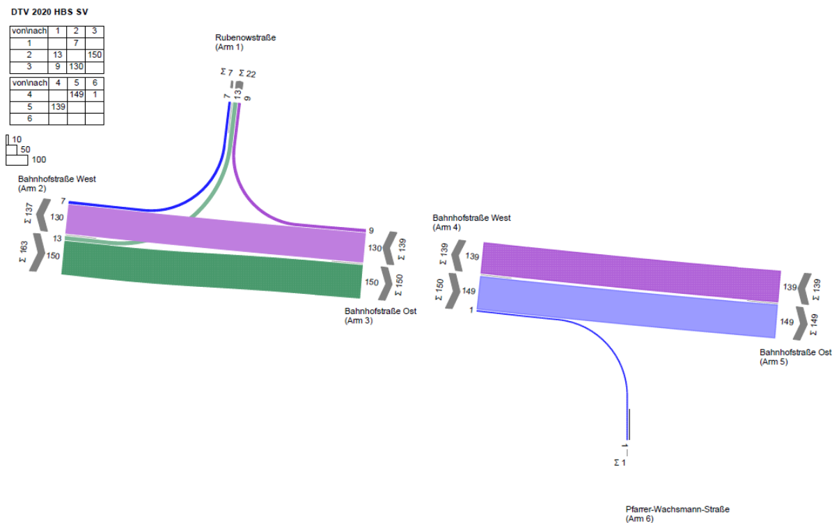
Abbildung 13 KP2 Bahnhofstr./Rubenowstr./Pfarrer-Wachsmannstr. – Hochrechnung DTV-SV [Kfz/24h]
