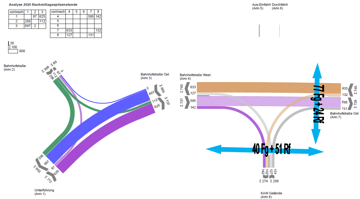
Abbildung 18 KP1 Bahnhofstraße/Zufahrt KAW – Nachmittagsspitzenstunde 16:15-17:15 [Kfz/h]
