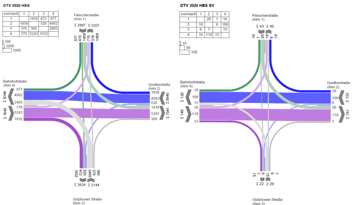
Abbildung 14 KP3 Bahnhofstr./Goethestr./Fleischerstr./Gützkower Str. DTV und DTV SV [Kfz/24h] DTV links, DTV SV rechts
