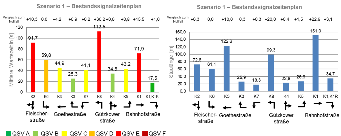
Abbildung 38 Leistungsfähigkeitsbewertung KP3 Bahnhofstr./Fleischerstr./Goethestr./Gutzkower Str. Prognoseplanfall 2030 – Signalzeitenplan signaltechnische Unterlagen
