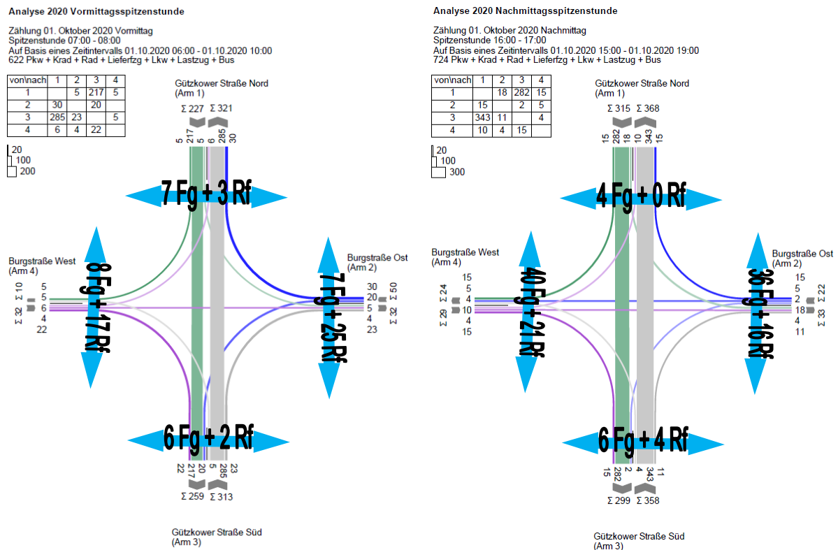
Abbildung 23 KP5 Gützkower Str./Burgstraße – Vor- und Nachmittagsspitzenstunde [Kfz/h]
