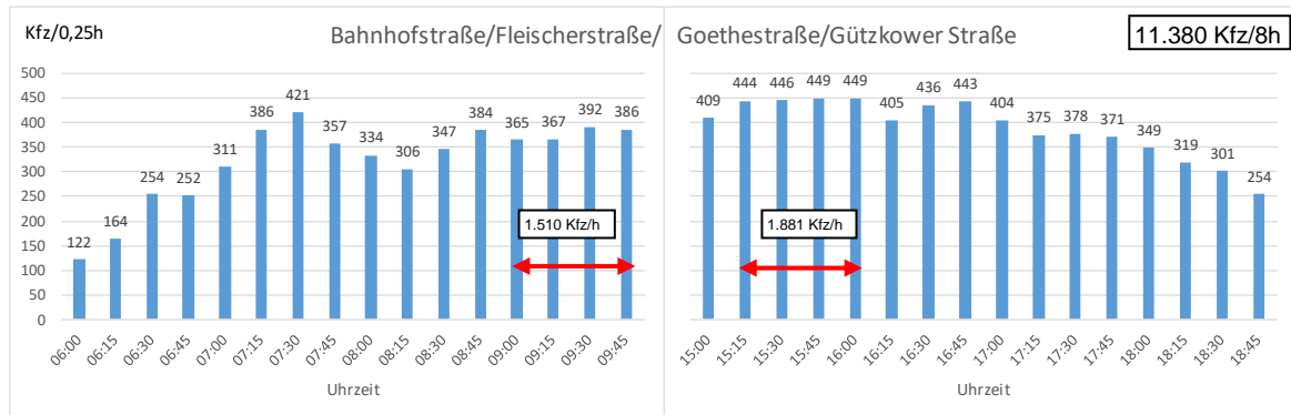
Abbildung 7 Tagesganglinie KP3 Bahnhofstr./Fleischerstr./Goethestr./Gützkower Str.KP4 Gützkower Straße/Wiesenstraße
