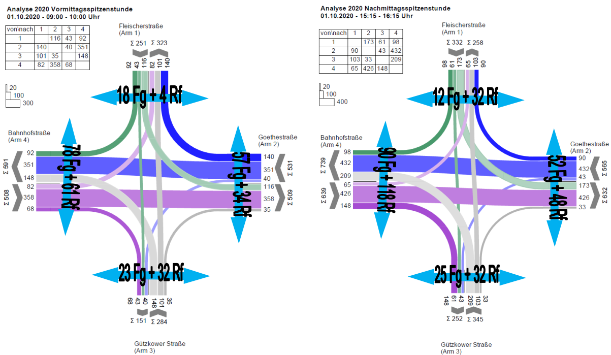
Abbildung 21 KP3 Bahnhofstr./Fleischerstr./Goethestr./Gützkower Str. – Vor- und Nachmittagsspitzenstunde [Kfz/h]
