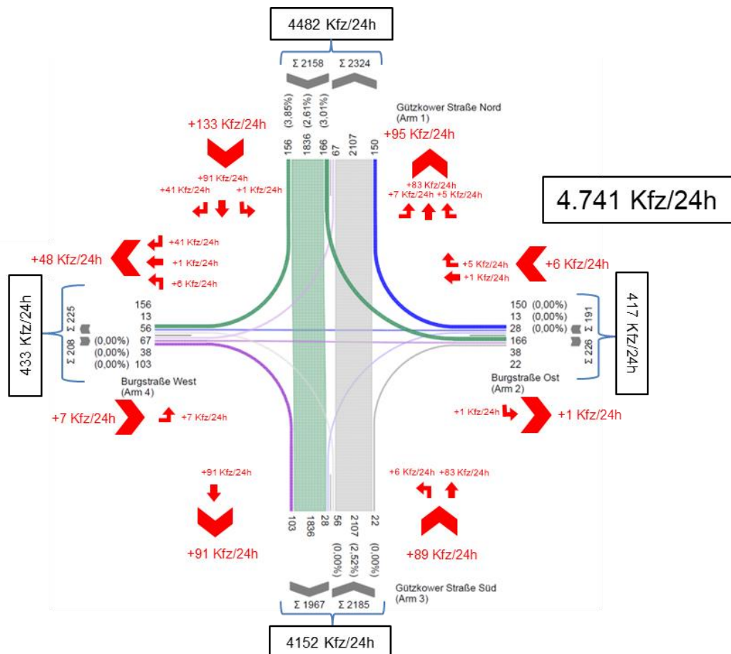
Abbildung 28 KP4 Gützkower Straße/Burgstraße Prognoseplanfall 2030 DTV [Kfz/24h]
