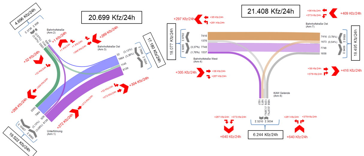
Abbildung 24 KP1 Bahnhofstraße/Zufahrt KAW-Gelände - Prognoseplanfall 2030 DTV [Kfz/24h]
