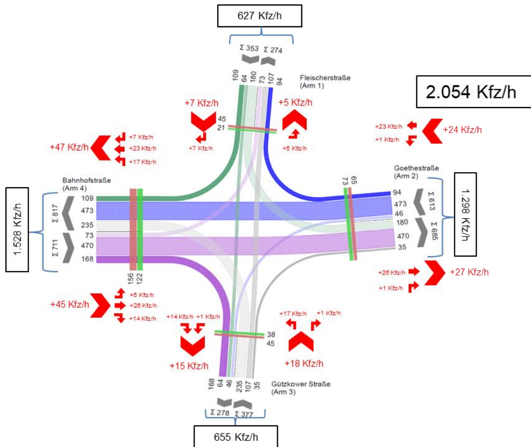
Abbildung 31 KP3 Bahnhofstr./Goethestr./Fleischerstr./Gützkower Str. Prognoseplanfall 2030 MSV [Kfz/h]
