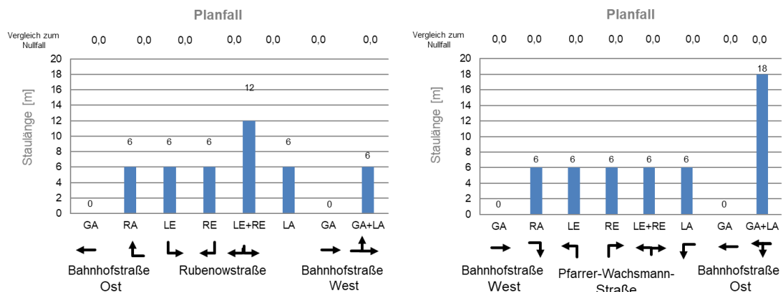
Abbildung 37 Stauraumlängen KP2 Bahnhofstr./Rubenowstr./Pfarrer-W.-Str. Prognoseplanfall 2030 kehrsstrom der Rubenowstraße mit 2 Aufstellplätzen und des Linksabbiegers in die Pfarrer-Wachsmann-Straße mit 3 Aufstellplätzen. Dabei ergeben sich keine Veränderung zum Null- und Analysefall.
