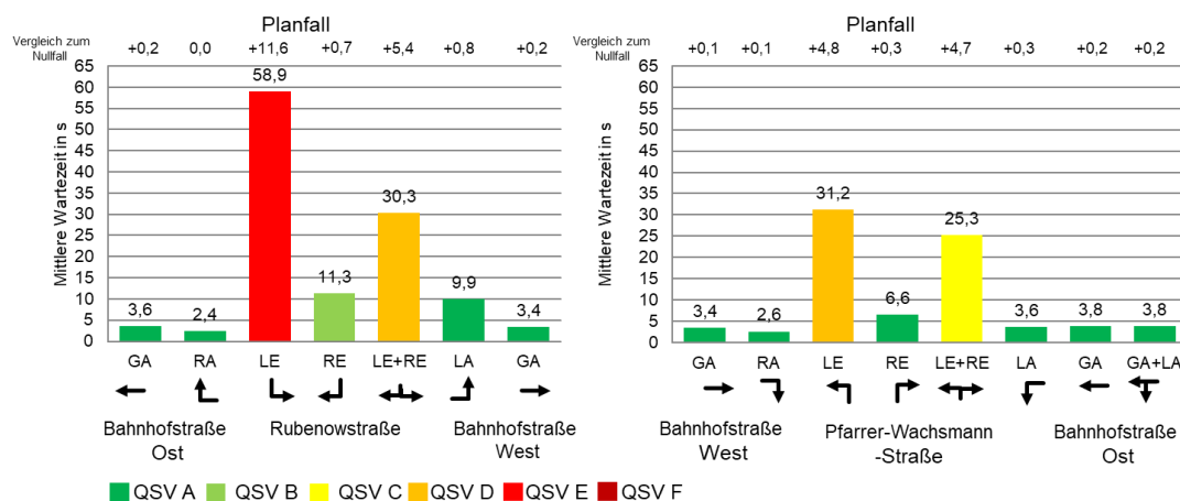
Abbildung 36 Leistungsfähigkeitsbewertung KP2 Bahnhofstr./Rubenowstr./Pfarrer-W.-Str. Prognoseplanfall 2030 Am Teilknoten 2 (Pfarrer-Wachsmann-Straße) wird die Gesamtqualitätsstufe QSV D erzielt. Der Grenzwert zur QSV C wird dabei relativ knapp verfehlt. Maßgebender Verkehrsstrom ist dabei der Linkseinbieger aus der Pfarrer-Wachsmann-Straße mit etwas über 31s. Alle anderen Verkehrsströme liegen unter 10s und erzielen die QSV A. Der Mischverkehrsstrom der Pfarrer-Wachsmann-Straße aus Links- und Rechtseinbiegern ist mit etwas über 25s in die Qualitätsstufe QSV C zu kategorisieren.
