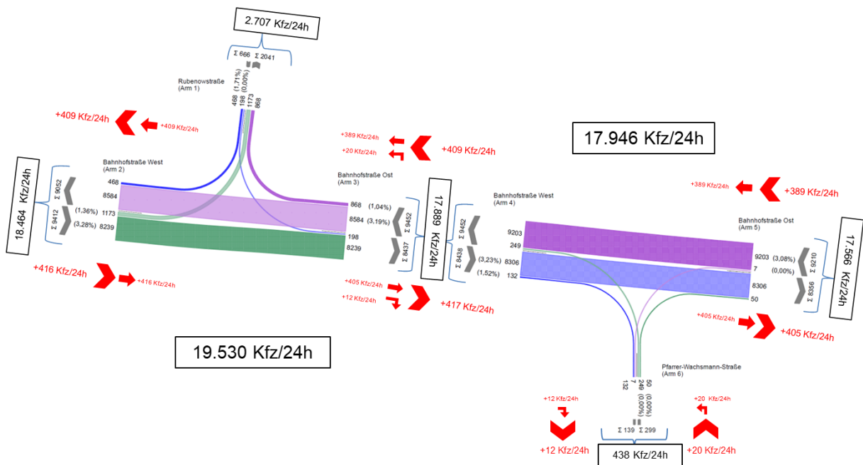
Abbildung 25 KP2 Bahnhofstr./Rubenowstr./Pfarrer-W.-Str. – Prognoseplanfall 2030 DTV [Kfz/24h]
