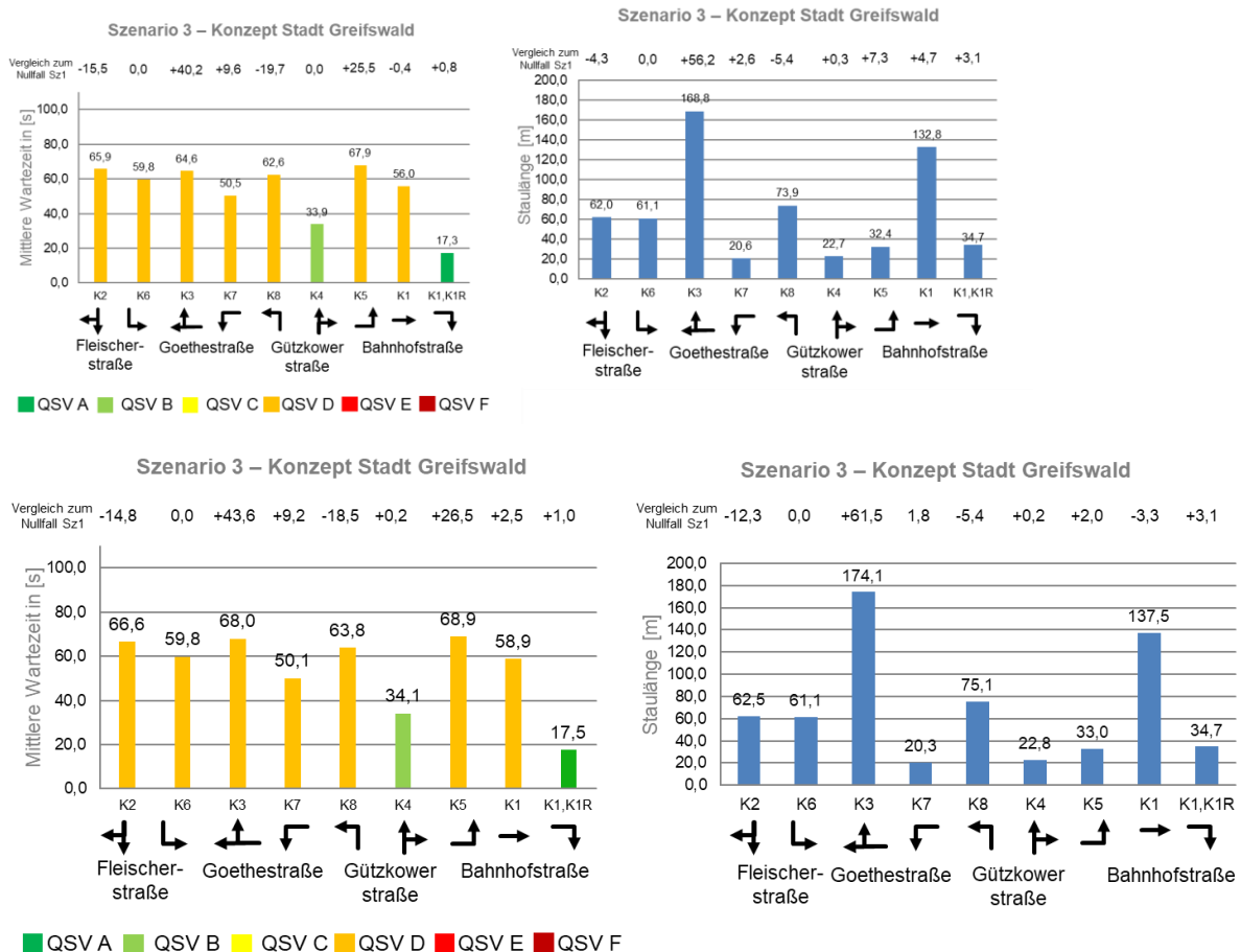
Abbildung 40 Leistungsfähigkeitsbewertung KP3 Bahnhofstr./Fleischerstr./Goethestr./Gützkower Str. Prognoseplanfall 2030 – Knotenpunktumgestaltung Konzept Stadt Greifswald
