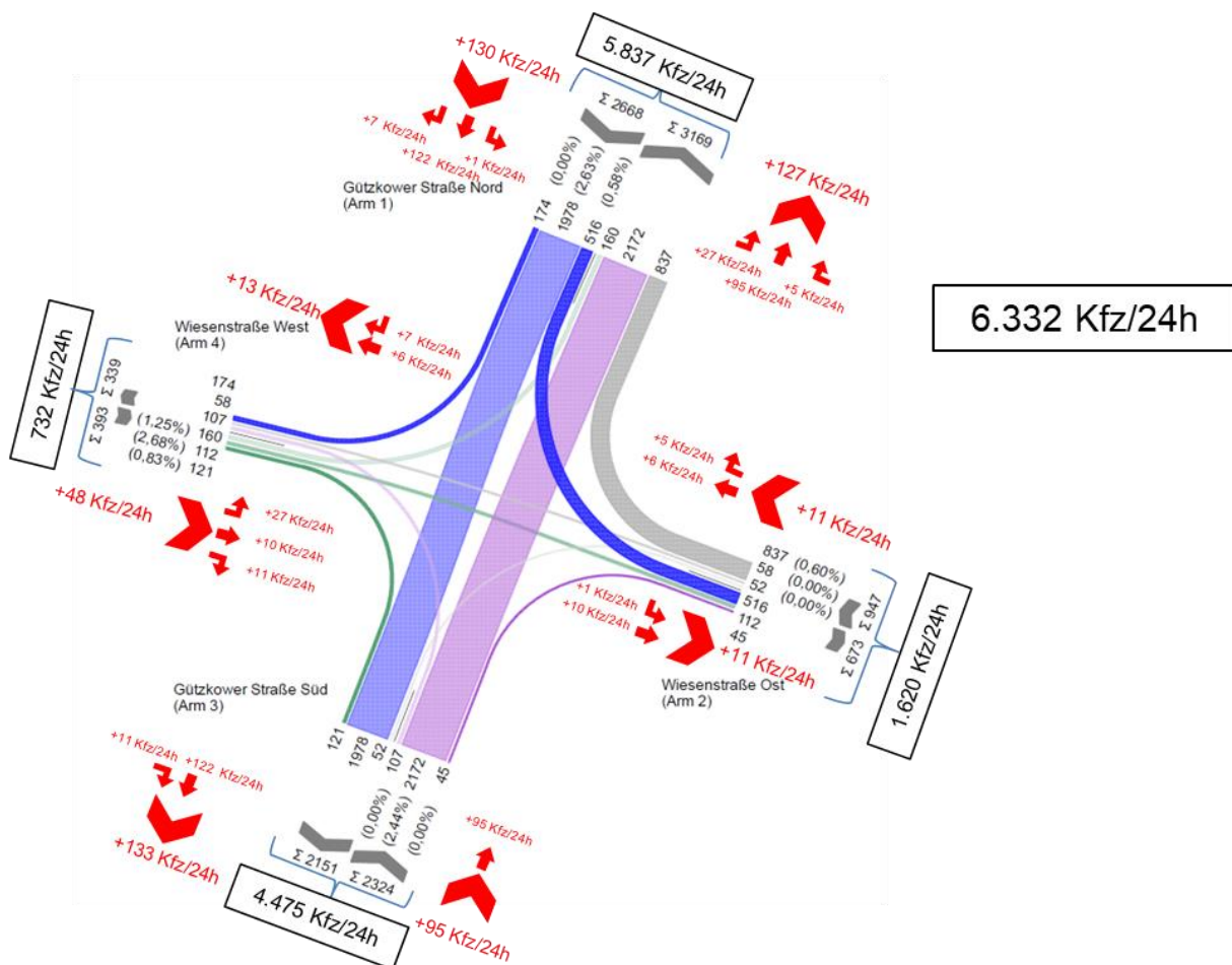
Abbildung 27 KP4 Gützkower Straße/Wiesenstraße Prognoseplanfall 2030 DTV [Kfz/24h]
