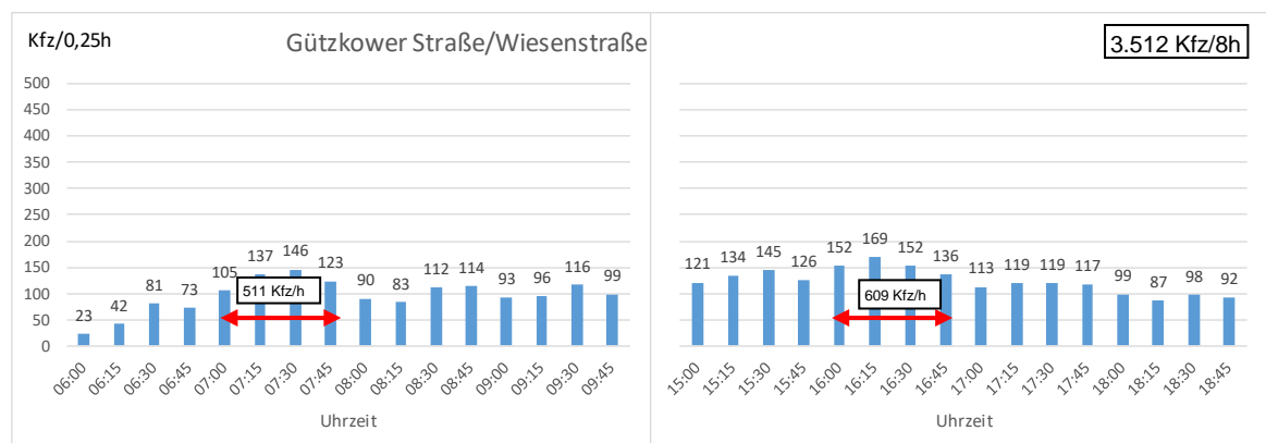
Abbildung 8 Tagesganglinie KP4 Gützkower Straße/Wiesenstraße
