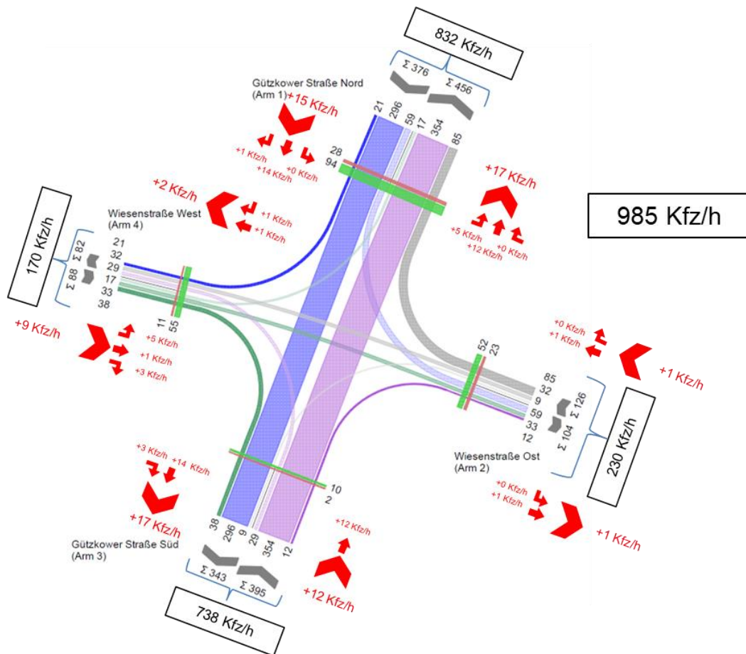
Abbildung 32 KP4 Gützkower Straße/Wiesenstraße Prognoseplanfall 2030 MSV [Kfz/h]
