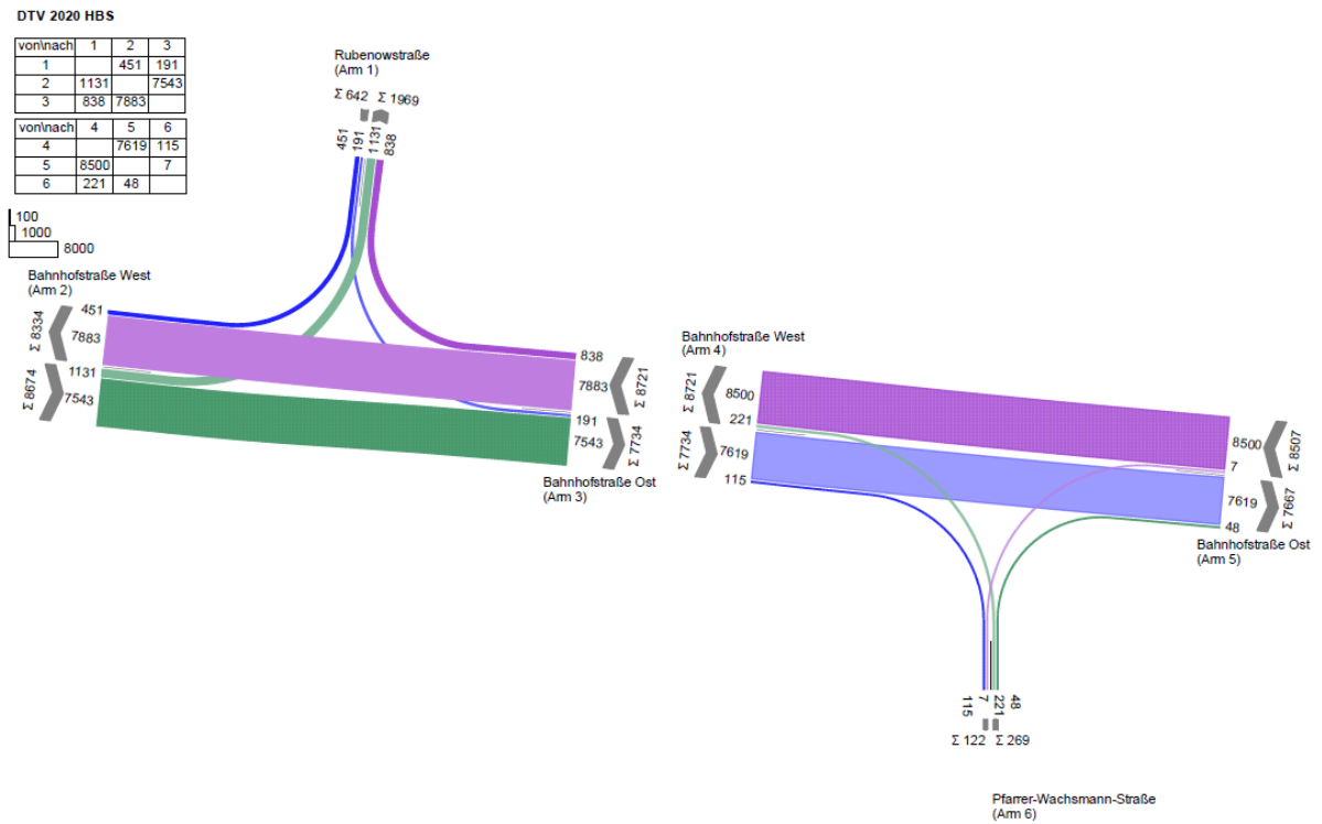
Abbildung 12 KP2 Bahnhofstr./Rubenowstr./Pfarrer-Wachsmann-Str. – Hochrechnung DTV [Kfz/24h]
