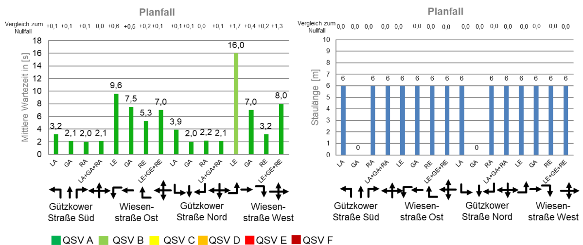
Abbildung 41 Leistungsfähigkeitsbewertung KP4 Gützkower Straße/Wiesenstraße Prognoseplanfall 2030
