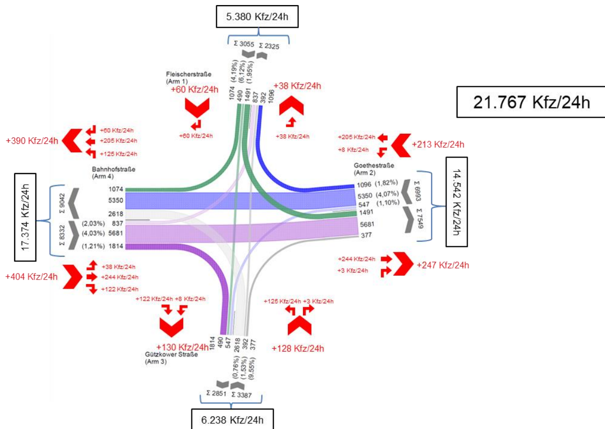
Abbildung 26 KP3 Bahnhofstr./Goethestr./Fleischerstr./Gützkower Str. Prognoseplanfall 2030 DTV [Kfz/24h]
