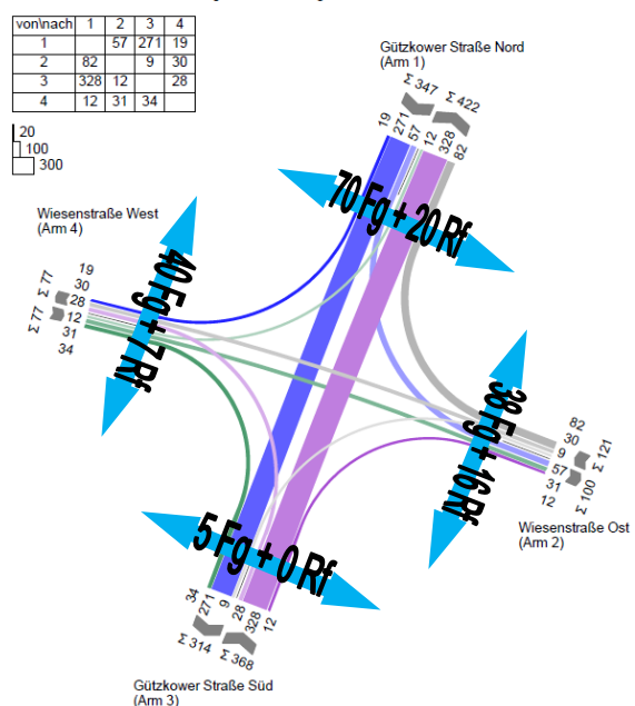
Abbildung 22 KP4 Gützkower Str./Wiesenstraße – Vor- und Nachmittagsspitzenstunde [Kfz/h]
