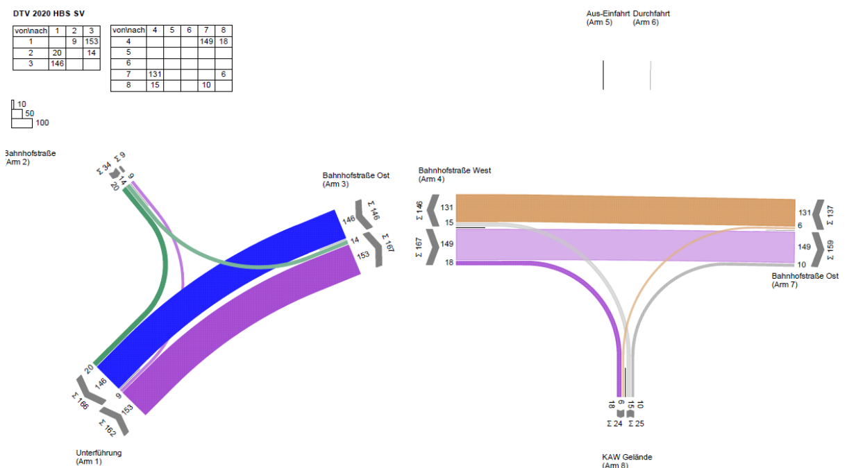
Abbildung 11 KP1 Bahnhofstraße/Zufahrt KAW-Gelände – Hochrechnung DTV SV [Kfz/24h]
