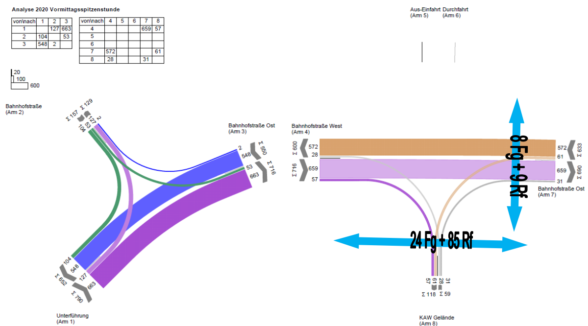
Abbildung 17 KP1 Bahnhofstraße/Zufahrt KAW – Vormittagsspitzenstunde 07:15-08:15 [Kfz/h]
