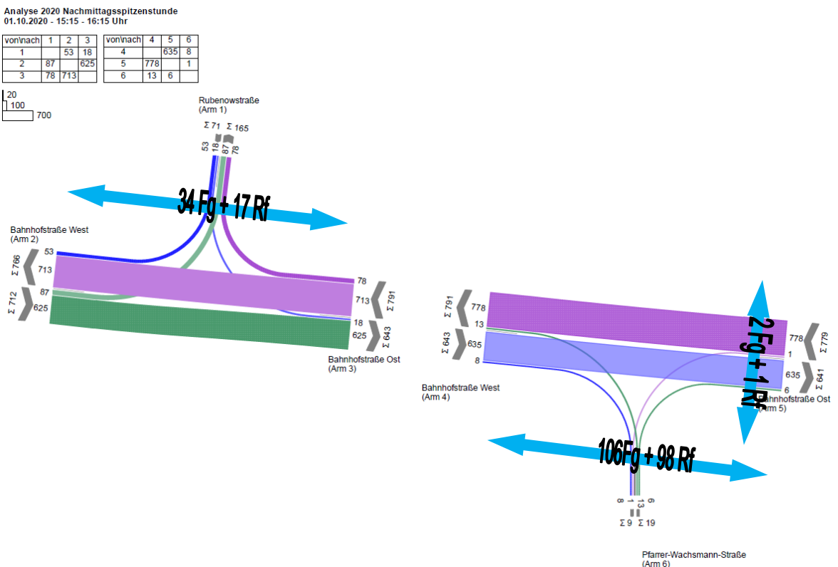
Abbildung 20 KP2 Bahnhofstr./Rubenowstr./Pfarrer-W.-Str – Nachmittagsspitzenstunde [Kfz/h]
