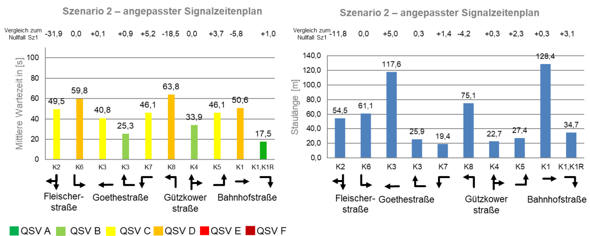
Abbildung 39 Leistungsfähigkeitsbewertung KP3 Bahnhofstr./Fleischerstr./Goethestr./Gützkower Str. Prognoseplanfall 2030 – modifizierter Signalzeitenplan auf Basis signaltechnische Unterlagen
