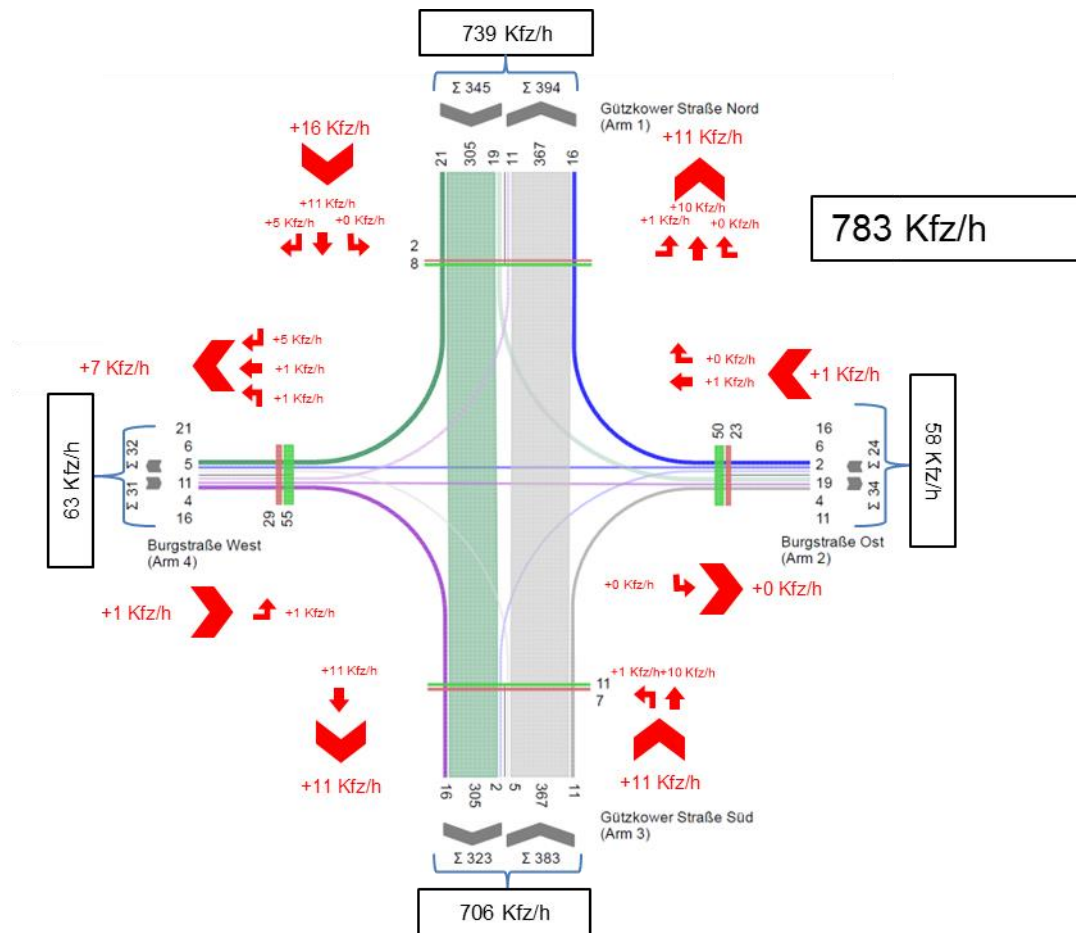
Abbildung 33 KP4 Gützkower Straße/Burgstraße Prognoseplanfall 2030 MSV [Kfz/h]
