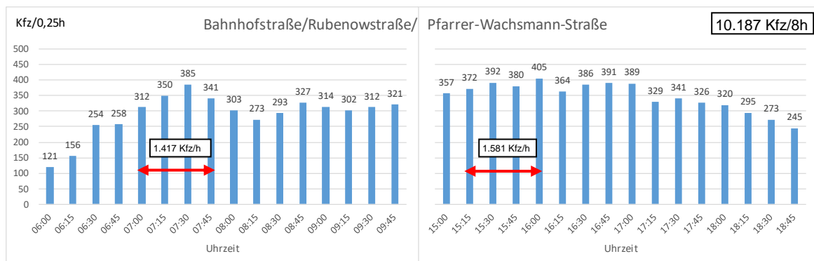
Abbildung 6 Tagesganglinie KP2 Bahnhofstraße/Rubenowstraße/Pfarrer-Wachsmann-Straße
