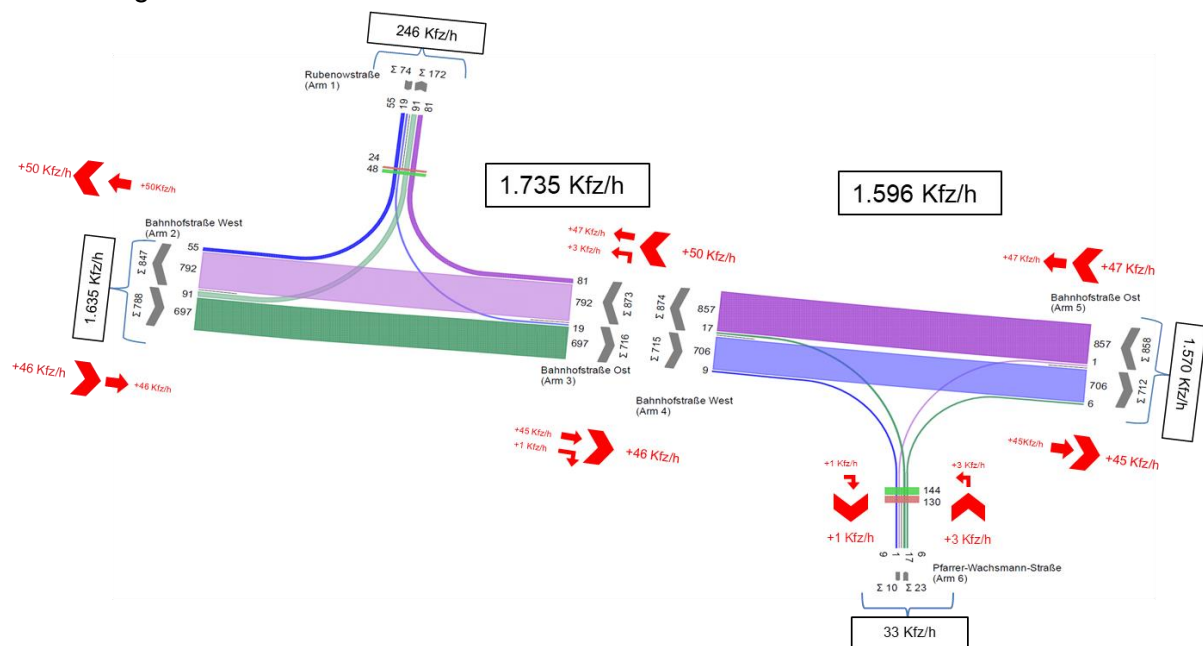
Abbildung 30 KP2 Bahnhofstr./Rubenowstr./Pfarrer-W.-Str. – Prognoseplanfall 2030 DTV [Kfz/h]
