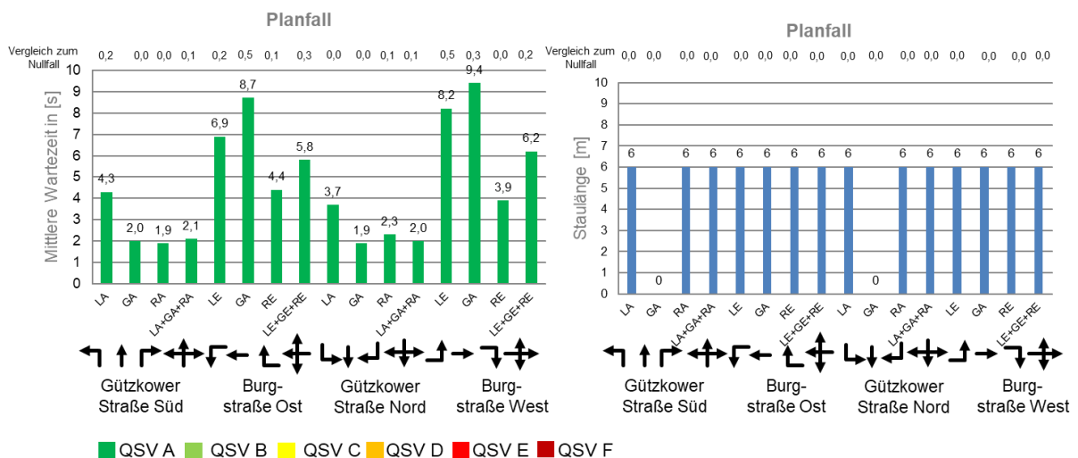
Abbildung 42 Leistungsfähigkeitsbewertung KP5 Gützkower Straße/Burgstraße Prognoseplanfall 2030
