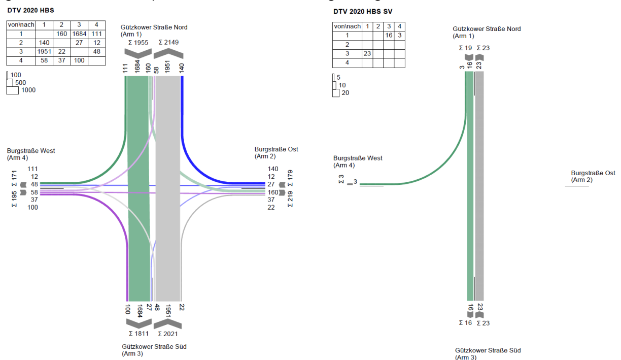
Abbildung 16 KP4 Gützkower Straße/Burgstraße DTV und DTV SV [Kfz/24h] DTV links, DTV SV rechts
