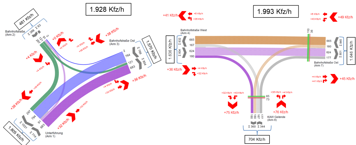
Abbildung 29 KP1 Bahnhofstraße/Zufahrt KAW-Gelände - Prognoseplanfall 2030 MSV [Kfz/h]
